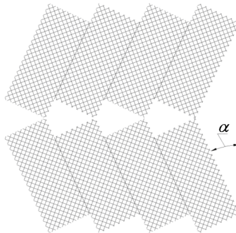
Рисунок 1. Блок оросителя состоящий из двух слоев
