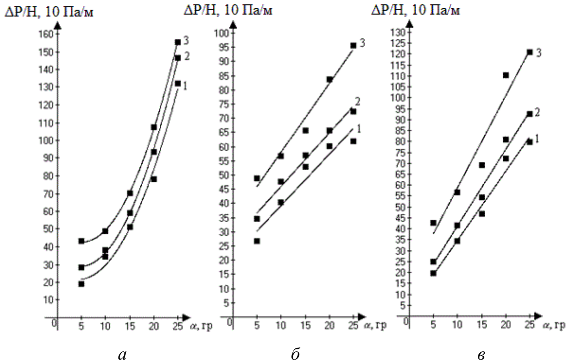
Рисунок 3. Зависимости удельного сопротивления орошаемых насадок от угла \alpha при скорости в расчете на полное сечения пустого аппарата - w_0 = 3 \frac{м}{с} : а – для насадки из сетки «M2», б – для насадки из сетки «Тип 3», в – для насадки из сетки «Ф4»; 1 – q_{ж} = 8 \text{ м}^3/(\text{м}^2 \cdot \text{ч}) , 2 – q_{ж} = 11,5 \text{ м}^3/(\text{м}^2 \cdot \text{ч}) , 3 – q_{ж} = 16 \text{ м}^3/(\text{м}^2 \cdot \text{ч})
