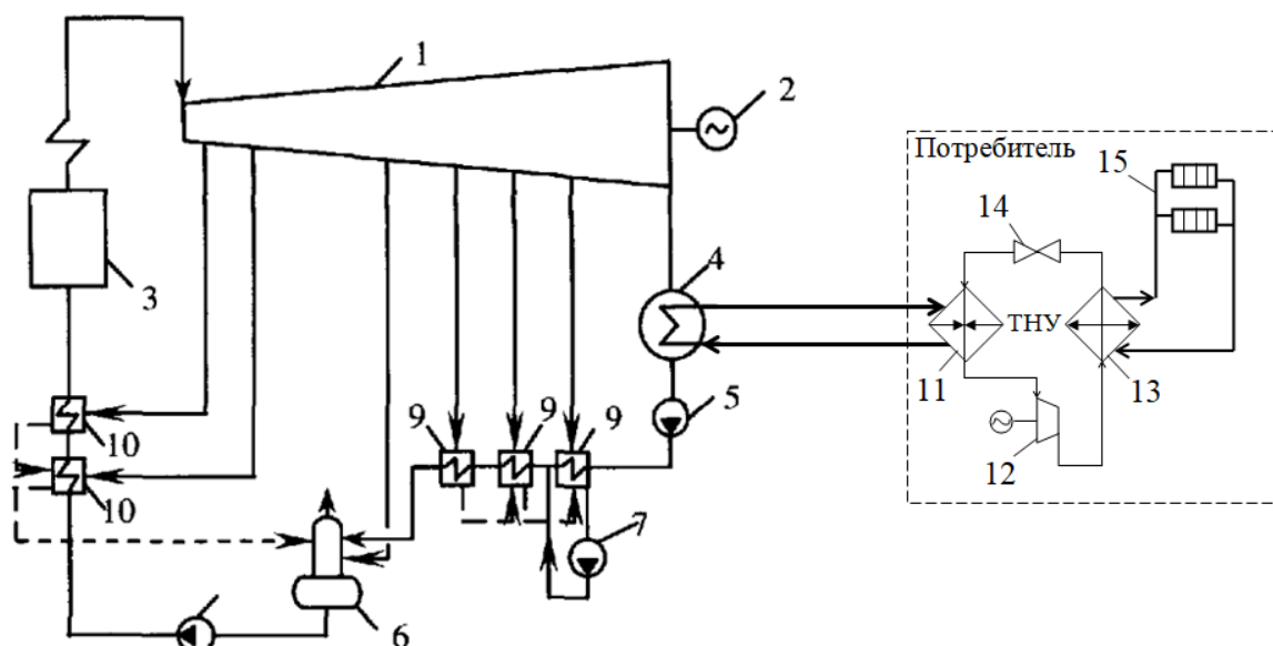
Рисунок 1 – Принципиальная схема системы теплоснабжения с ТНУ: 1 – конденсационная турбина, 2 – электрогенератор, 3 – энергетический котел, 4 – конденсатор ПТУ, 5 – конденсатный насос, 6 – деаэратор, 7 – конденсатный насос регенеративных подогревателей, 8 – питательный насос, 9 – ПНД, 10 – ПВД, 11 – испаритель, 12 – компрессор, 13 – конденсатор ТНУ, 14 – дросселирующий вентиль, 15 – индивидуальная система отопления
