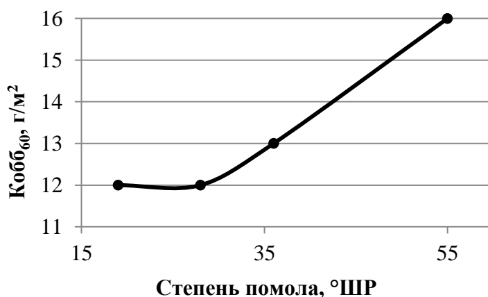
Рисунок 7 - График изменения степени проклейки от времени размола для СФАЛБ
