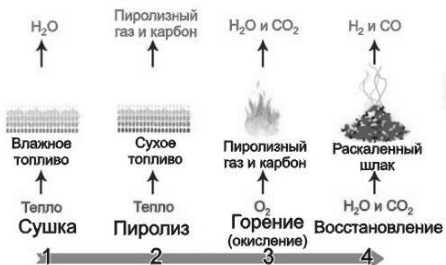
Рисунок 1 – Принципиальная схема пиролиза
