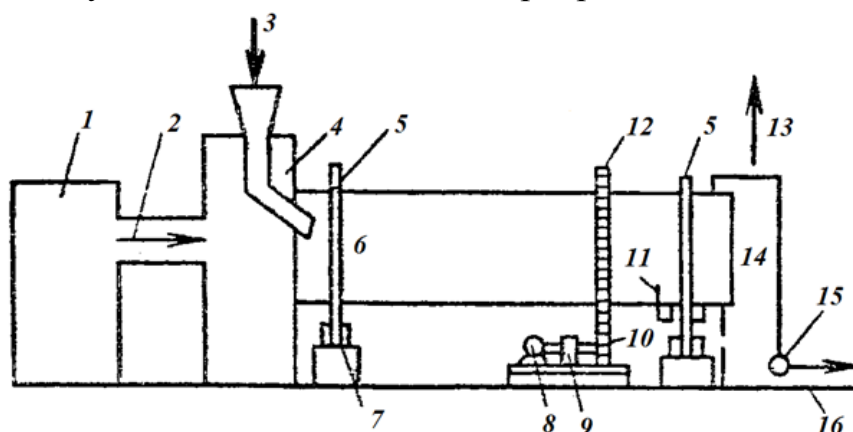
Рисунок 1 - Схема барабанной сушильной установки: 1 – топка; 2 – топочные газы; 3 – подача кека; 4 – загрузочная камера; 5 – бандаж; 6 – барабан; 7 – опорные ролики; 8 – электродвигатель; 9 – редуктор; 10 – ведущая шестерня; 11 – упорные ролики; 12 – зубчатый венец; 13 – отработавшие газы; 14 – выгрузочная камера; 15 – шлюзовый затвор; 16 – выпуск сухого осадка
