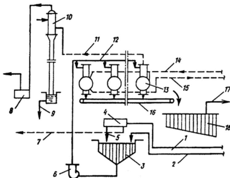
Рисунок 2 – Технологическая схема вакуум-сушки осадков: 1 – уплотненный избыточный активный ил; 2 – сырой осадок из первичных отстойников; 3 – резервуар-смеситель; 4 – центрифуга; 5 – центрифугированный активный ил; 6 – насос для подачи осадка в сушилку; 7 – фугат в аэротенки; 8 – вакуум-насос; 9 – конденсат вторичного пара; 10 – барометрический конденсатор; 11 – вторичный пар в конденсатор; 12 – исходный осадок в сушилки; 13 – вакуум-сушилки; 14 – пар от котельной; 15 – конденсат в котельную; 16 – конвейер сухого осадка; 17 – сухой осадок; 18 – бункер сухого осадка
