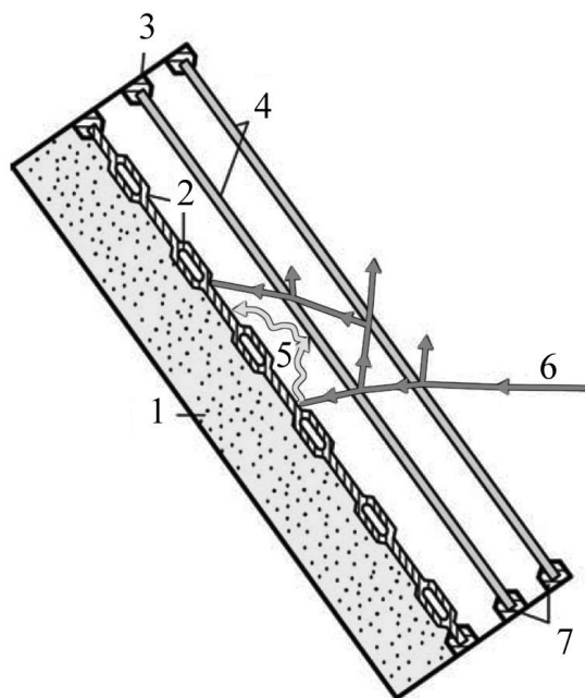
Рисунок 1 – Схема "плоского" солнечного коллектора: 1 – изоляция; 2 – лучевоспринимающая поверхность; 3 – кожух; 4 – стекло; 5 – излучение лучевоспринимающей пластины; 6 – солнечные лучи; 7 – уплотнитель
