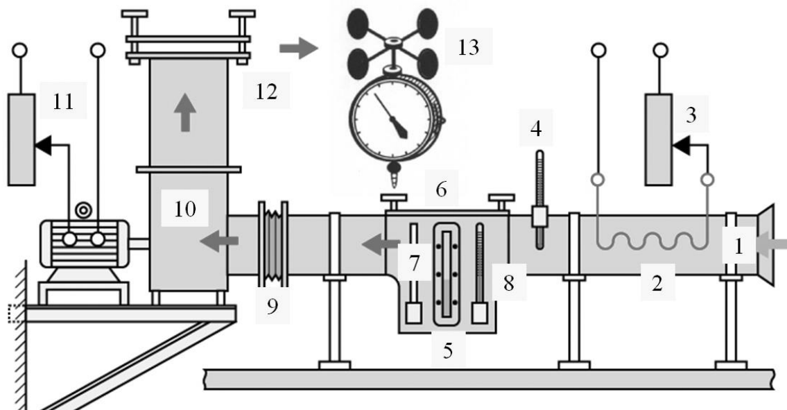
Рисунок - 1. Схема экспериментальной установки: 1 - аэродинамическая труба; 2 - нагреватель; 3 - ЛАТР для нагревателя; 4 - термометр для измерения температуры воздуха; 5 - рабочая камера; 6 - крышка камеры; 7 - водоуказательное стекло; 8 - термометр для измерения температуры воды; 9 - брезентовая вставка; 10 - центробежный вентилятор; 11 - ЛАТР для вентилятора; 12 - регулирующая заслонка; 13 - анемометр цифровой
