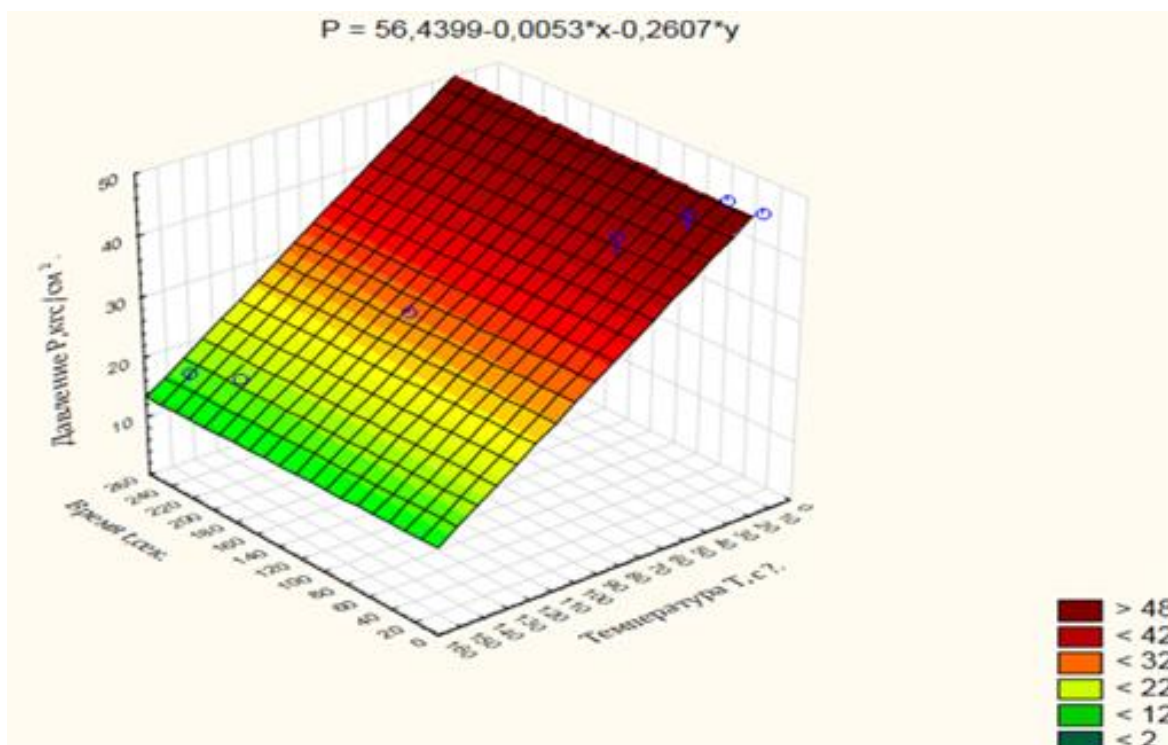
Рисунок 2 – Зависимость давления прессования от времени и температуры нагрева матрицы
