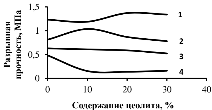
Рисунок 2 – Влияние процентного содержания полиядерных комплексов алюминия и цеолита на предел прочности
