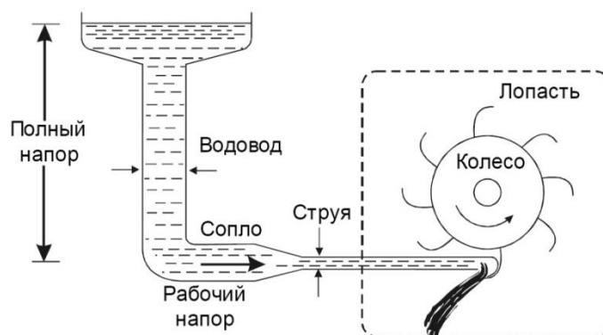
Схема работы активной турбины Пелтона
