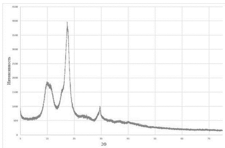
Рисунок 1 - Рентгенограмма исходной МКЦ
