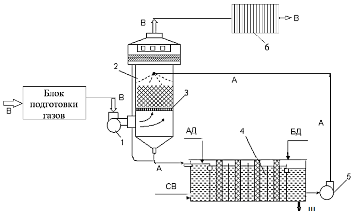
Рисунок 2 – Схема комбинированной очистки низкоконцентрированных выбросов от дурнопахнущих веществ: 1 – вентилятор; 2 – абсорбер (скруббер); 3 – массообменная решетка; 4 – биореактор; 5 – насос, 6 – фильтр; А – циркулирующий абсорбент; В–вентиляционный воздух; АД – абсорбент; БД – биогенные добавки; СВ – сжатый воздух, Ш – шлам
