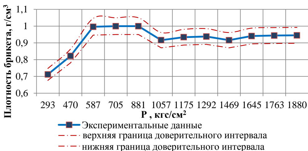
Рисунок 1 – Зависимость плотности брикета от давления прессования
