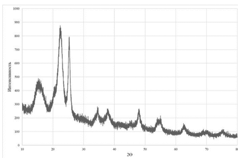
Рисунок 3 - Рентгенограмма нанокompозита МКЦ – оксида титана
