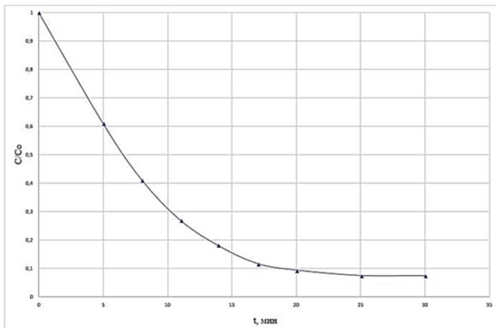
Рисунок 5 - Кинетика фотокаталитического окисления метиленового голубого под действием нанокompозита МКЦ – TiO 2 : C 0 – исходная концентрация красителя, C – концентрация красителя в процессе разложения
