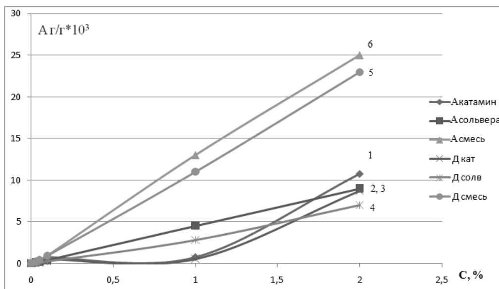
Зависимость адсорбции-десорбции ПАВ целлюлозой от концентрации ПАВ в растворе
