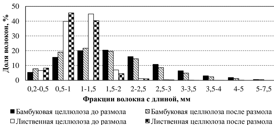
Рисунок 3 - Характеристики фракций волокна бамбуковой и лиственной целлюлозы: фракционный состав по длине волокна
