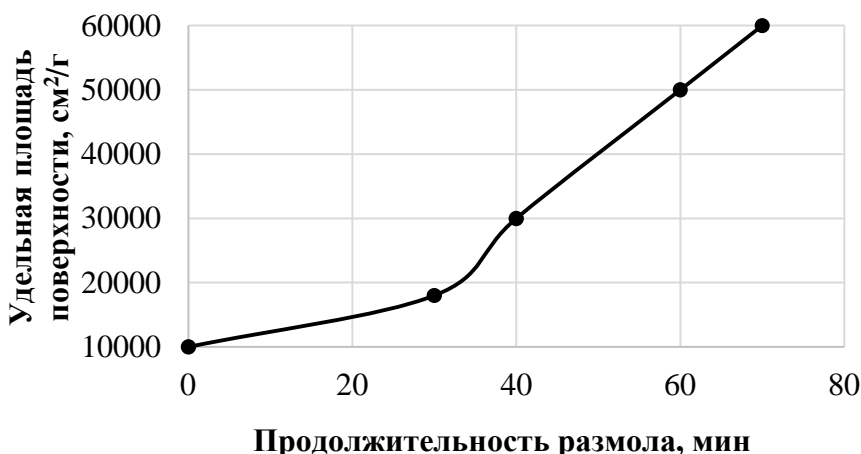
Рисунок 2- Кривая изменения удельной площади поверхности целлюлозы в процессе размола в зависимости от его продолжительности
