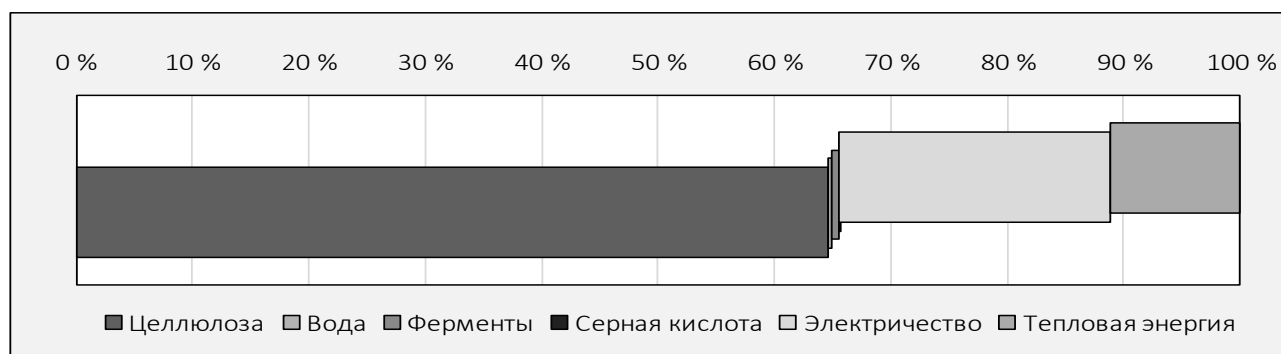
Рисунок 3 - Удельное влияние входящих потоков, требуемых для производства наноцеллюлозы методом HefCel
