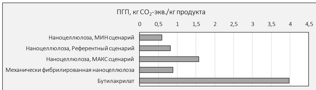
Рисунок 4 – Вклад в глобальное потепление производств nanoцеллюлоз, изготовленных различными методами, и бутилакрилата
