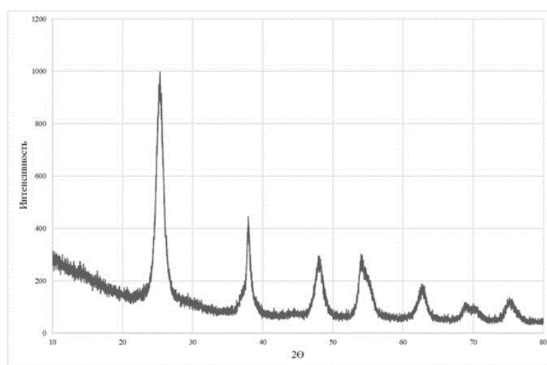
Рисунок 2 - Рентгенограмма наночастиц оксида титана
