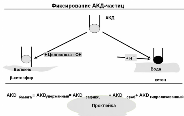
Рисунок 4 - Схема процесса проклейки бумаги и картона клеями на основе АКД
