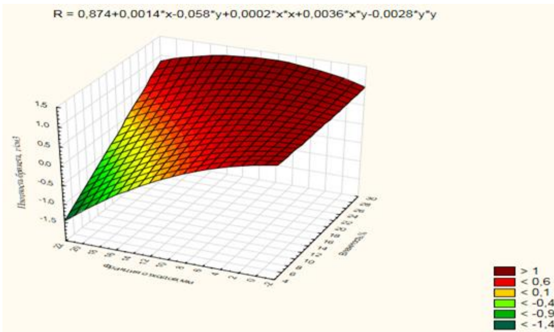
Рисунок 3 – Зависимость плотности брикета от влажности и фракционного состава
