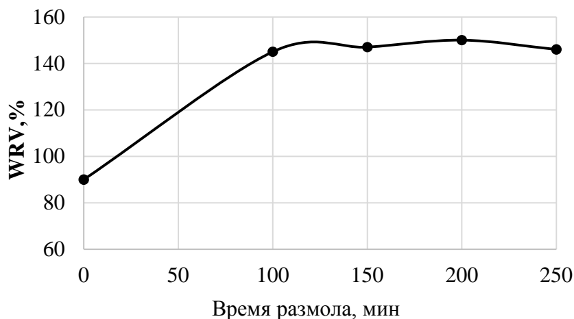
Рисунок 3 - Изменение водоудержания от времени размола
