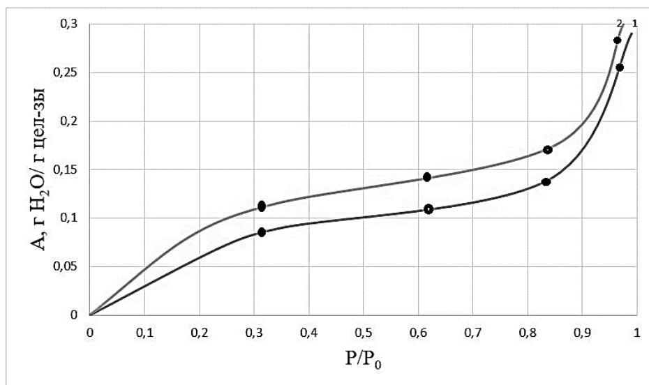
Рисунок 4 – Изотермы сорбции паров воды: 1 – кривая сорбции МКЦ, 2 – кривая сорбции гибрида МКЦ – TiO 2
