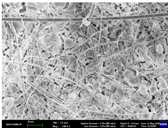
Рисунок 1 – Микрофотография структуры композитного материала на основе стеклянных волокон
