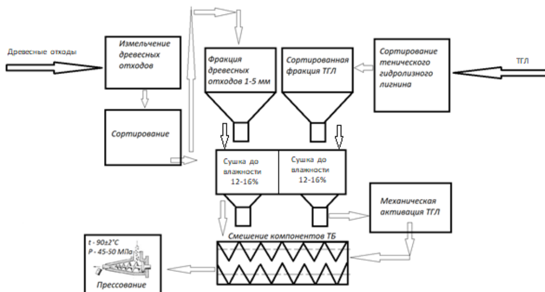
Рисунок 4 – Инновационная схема производства топливных брикетов из лесосырьевых ОТХОДОВ
