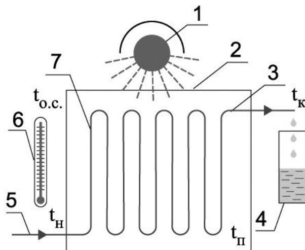
Рисунок 2 – Схема установки: 1 – лампа (имитирующая солнце); 2 – кожух коллектора; 3 – слив воды из коллектора; 4 – мензурка; 5 – подача воды в коллектор; 6 – термометр; 7 – трубки коллектора
