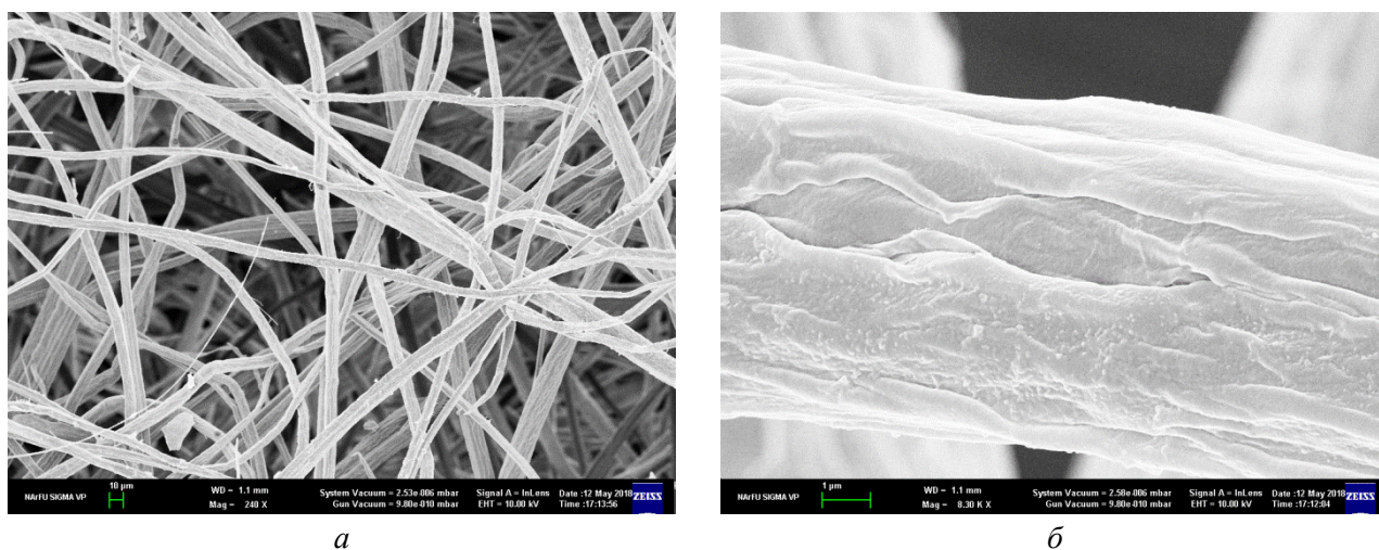
Рисунок 1 - Микрофотографии образцов бамбуковой целлюлозы (получены на электронном микроскопе Zeiss SIGMA VP): а – волокна; б – поверхность волокна
